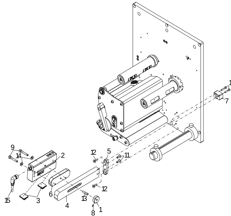
rechte Ausführung right version
