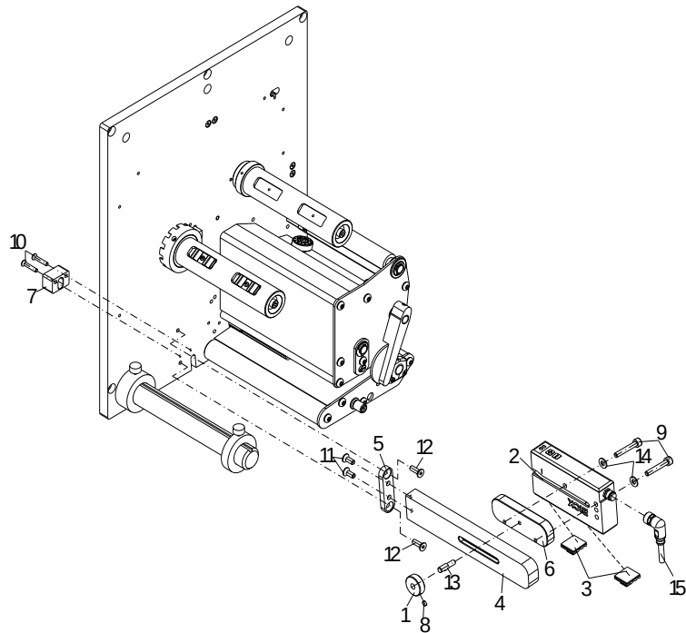
linke Ausführung left version
